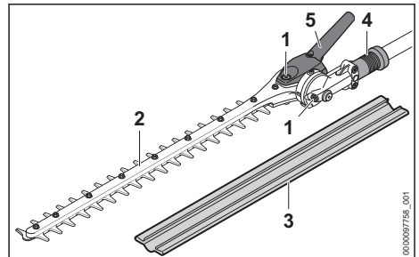
Verstellbares Schneidmesser
